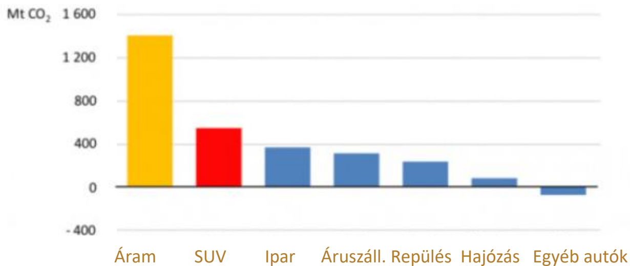
CO 2 kibocsátás változás szektoronként 200-2018
